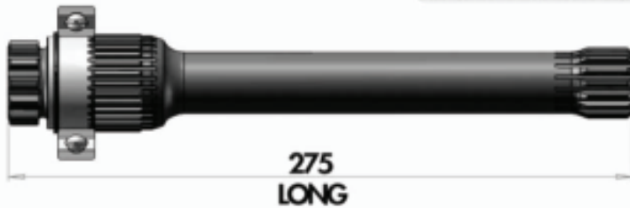
Mercedes Actros (G 125-135-155-180-200 210-221-240-255-260)
